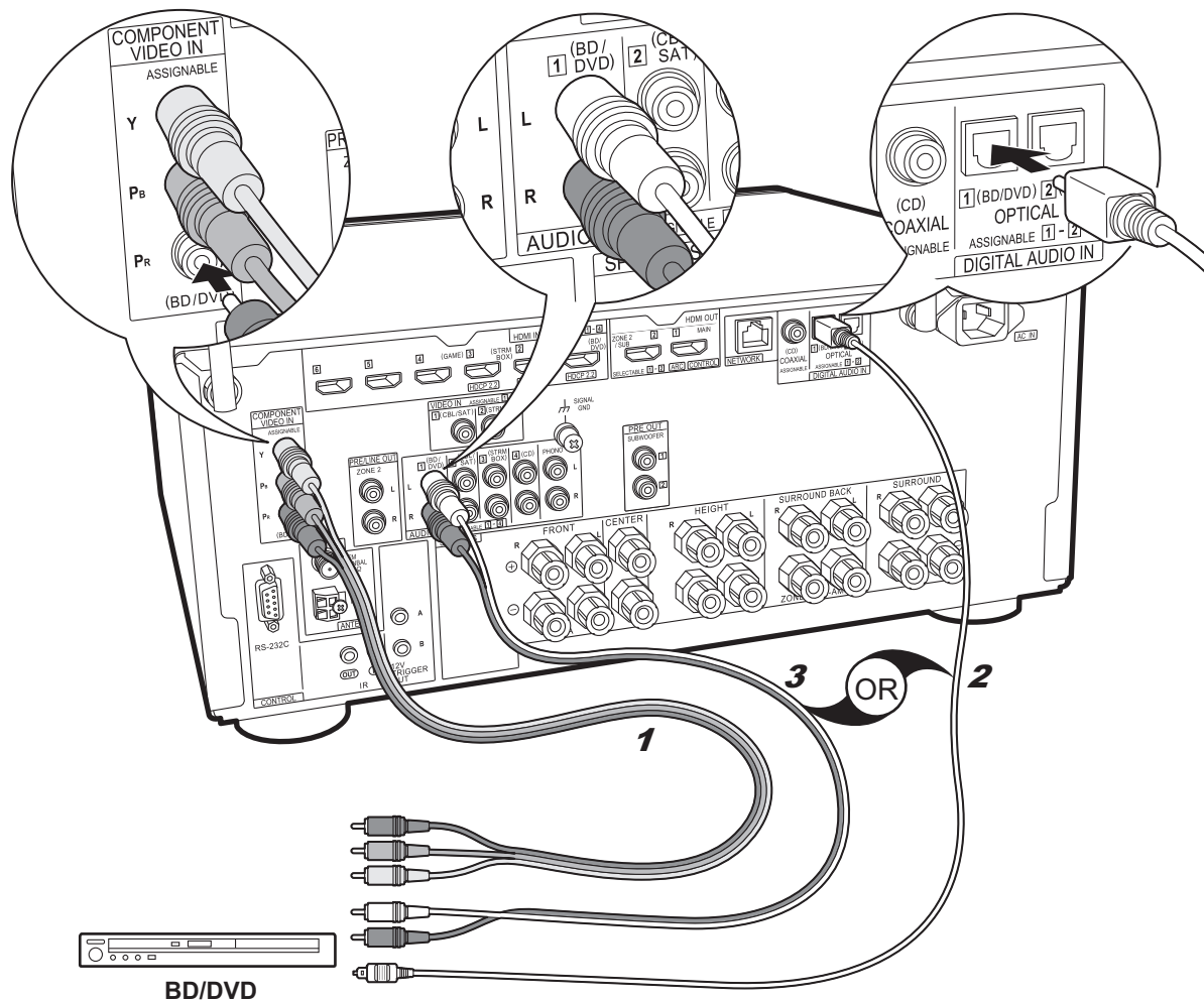
1 Компонентный видеокабель, 2 Цифровой волоконно-оптический кабель, 3 Аналоговый аудиокабель
